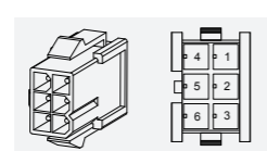
动力侧线缆6PIN接插件
